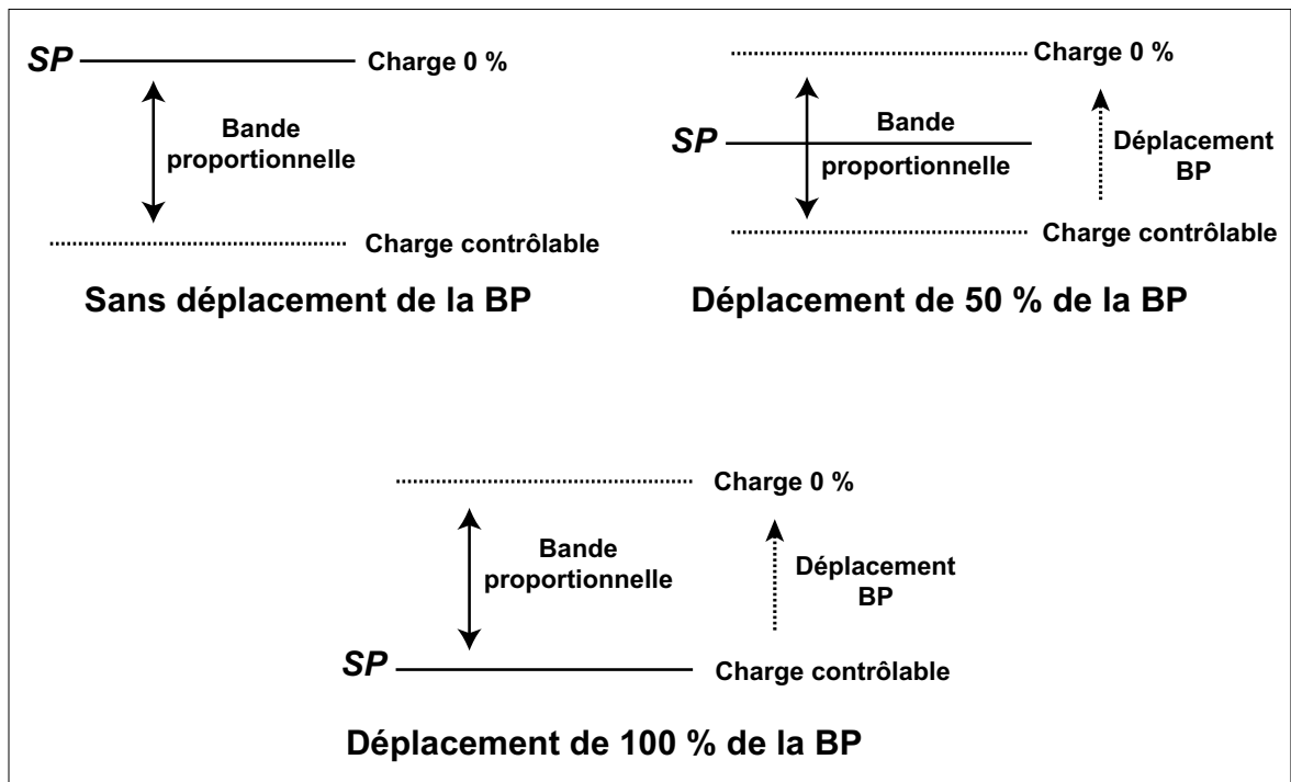
Figure 8.9 Déplacement de la bande proportionnelle en mode d'action inverse
