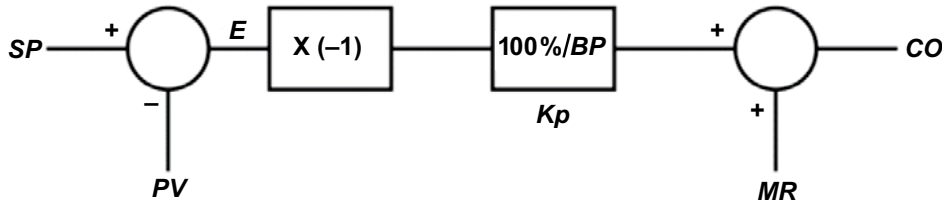
Figure 8.8 Régulateur à action directe avec MR (valeur de soutien)
