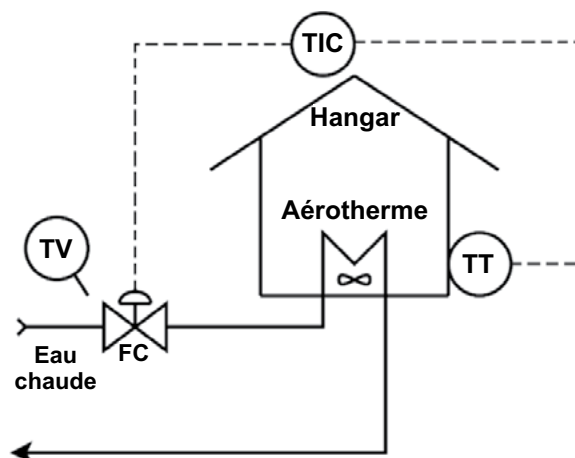
Figure 8.3 Bande proportionnelle en mode d'action inverse
