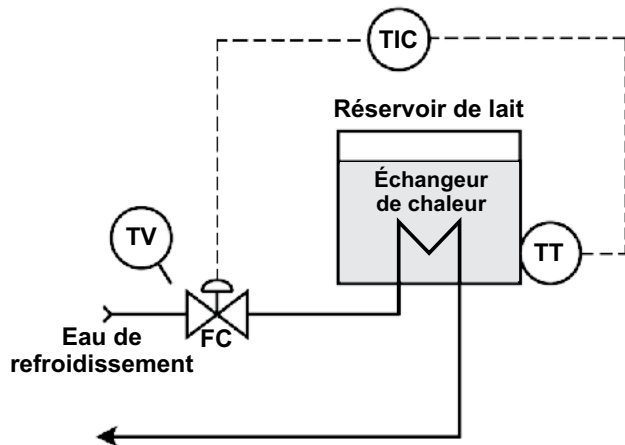
Figure 8.1 Système avec un régulateur à action directe
