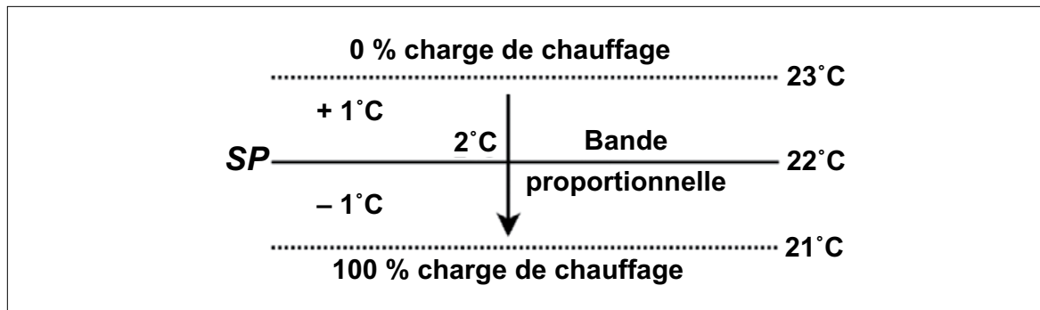
Figure 8.5 Bande proportionnelle déplacée en mode d'action inverse
