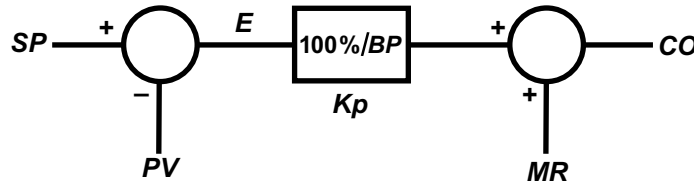
Figure 8.10 Régulateur à action inverse avec MR (valeur de soutien)
