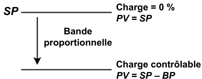
Figure 8.4 Bande proportionnelle en mode d'action inverse sans valeur de soutien
