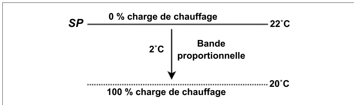
Figure 8.6 Bande proportionnelle non déplacée en mode d'action inverse
