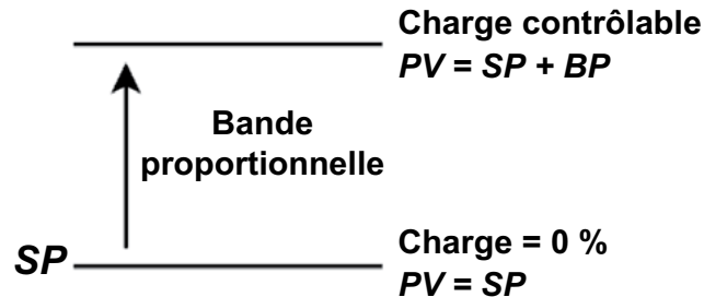
Figure 8.2 Bande proportionnelle en mode d'action directe sans valeur de soutien
