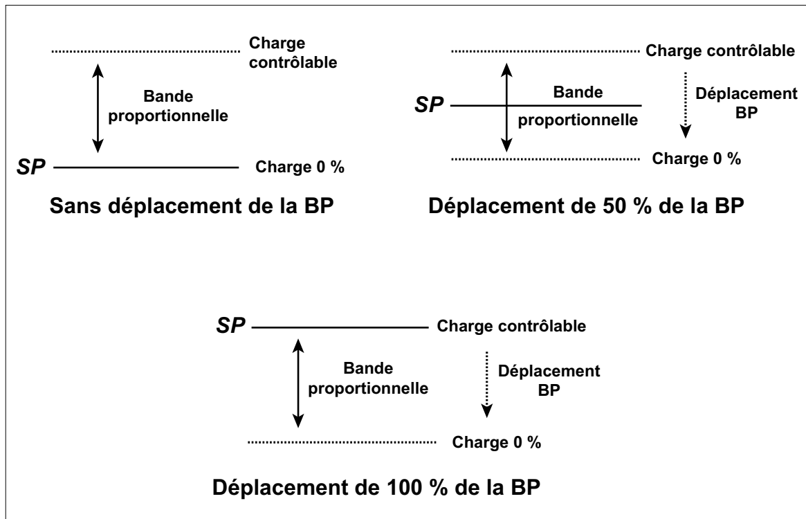
Figure 8.7 Déplacement de la bande proportionnelle en mode d'action directe
